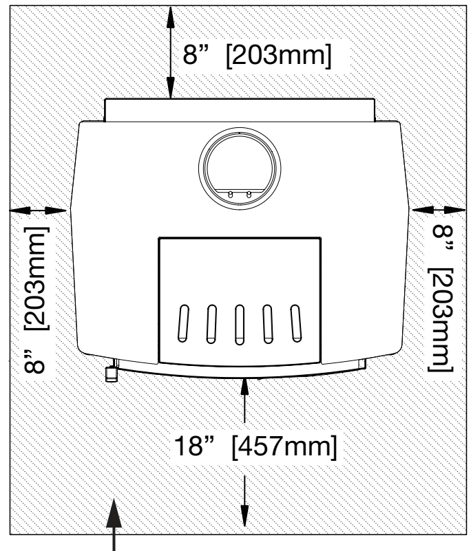
Non - combustible floor protector
